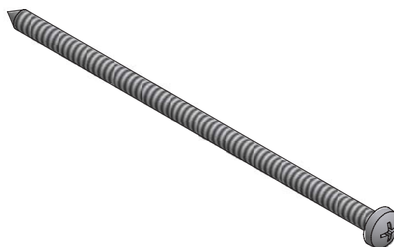
Blechschraube ISO 7049, 4,2 x 100
