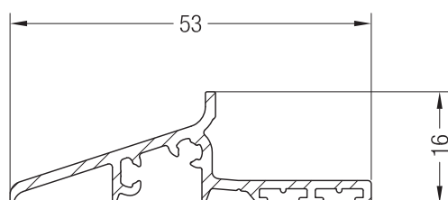
Wetterschenkel SYNEGO®
