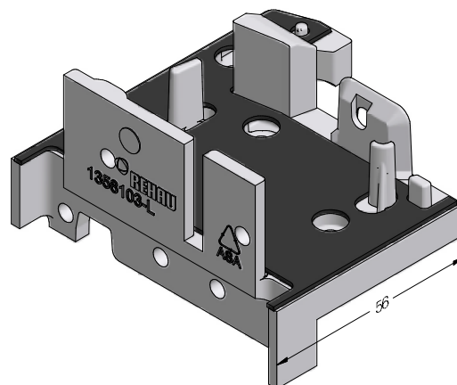
Schwellenhalter Blendrahmen 82 SYNEGO®
