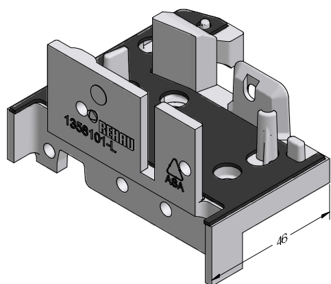
Schwellenhalter Blendrahmen 72 SYNEGO®
