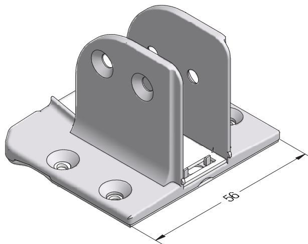
Mechanischer Verbinder Sprosse 68 SYNEGO®
